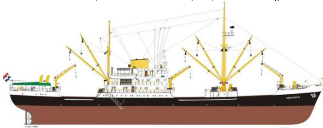
ms Van Neck (III) bjr 1955 Boele's scheepsw.& mach.fabr: tekening Robert Bersma
